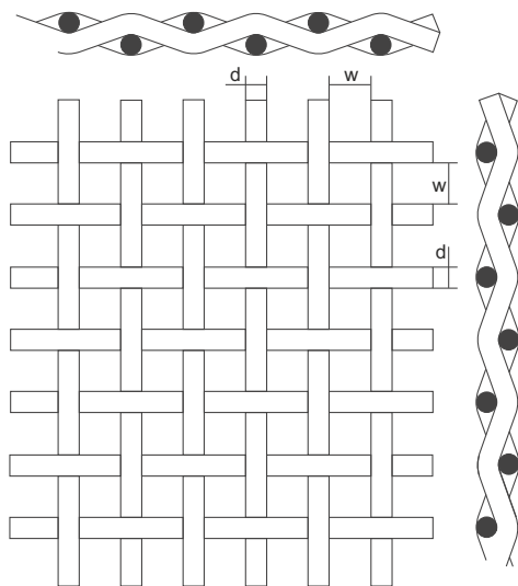
Рисунок 1. Прямое переплетение
